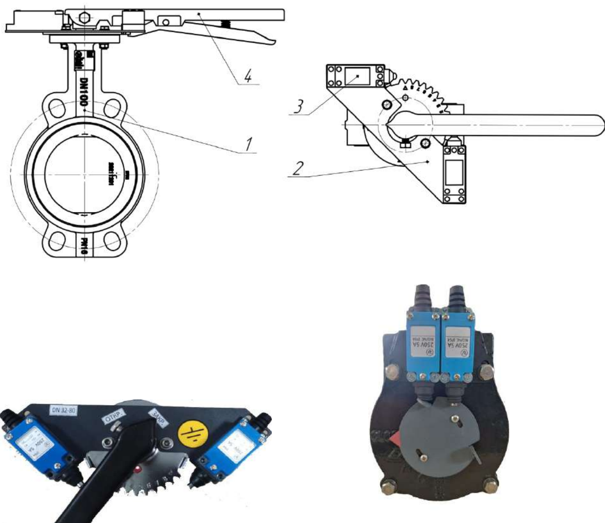
Общий вид УКП на затворе Ridval тип RVB 01 и редукторе.
